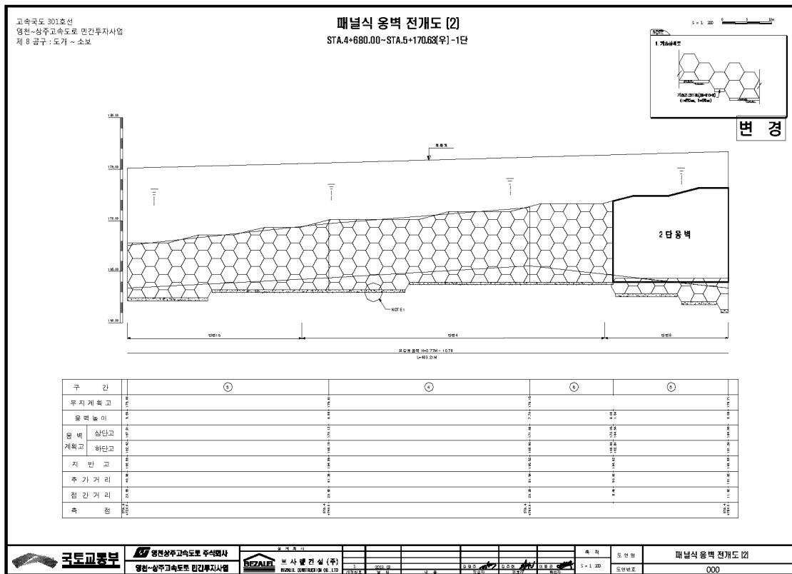
【그림 1.1.3】 전개도
