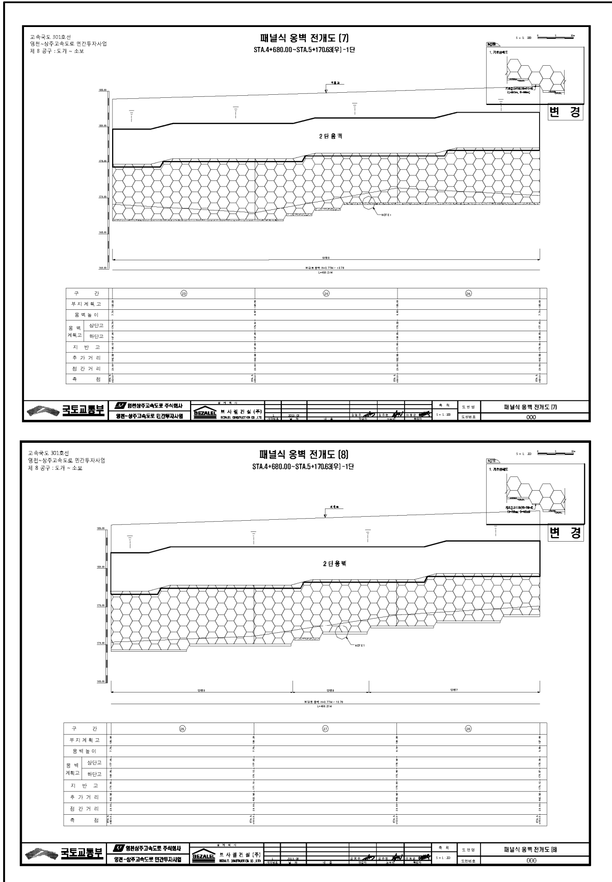
【그림 1.1.3】전개도(계속)
