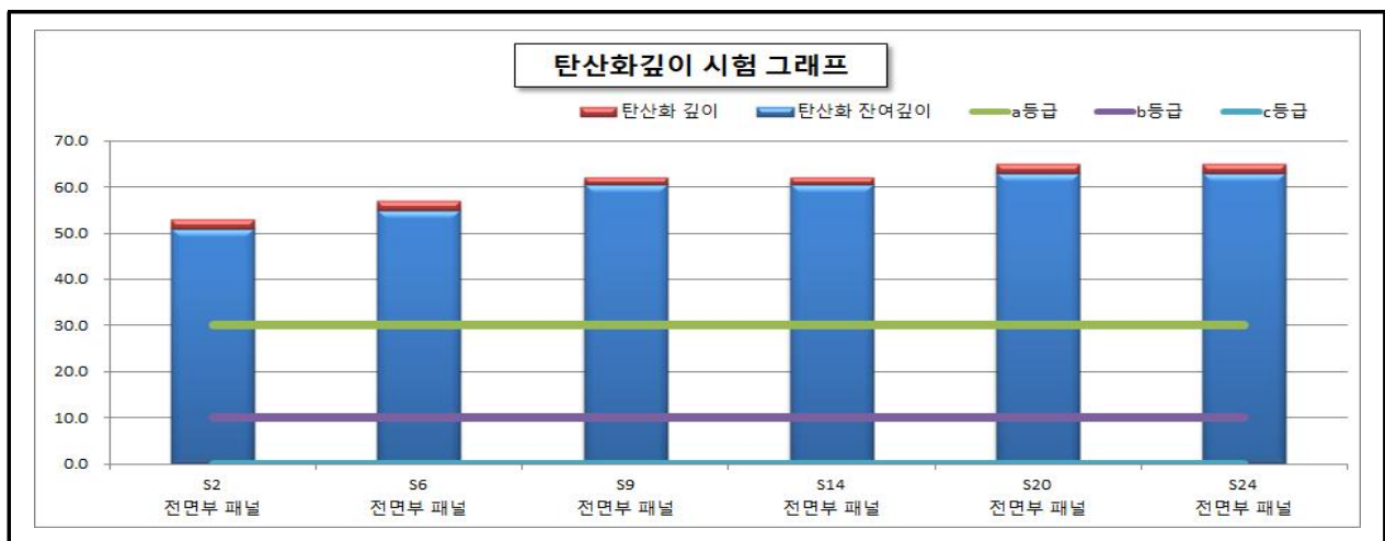
【그림 1.4.3】 탄산화 깊이 측정결과
