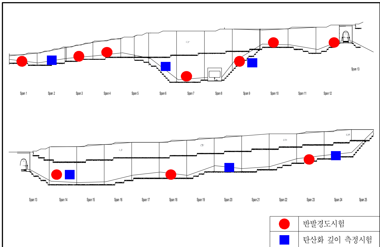
【그림 1.4.1】 콘크리트 재료시험 조사 위치도
