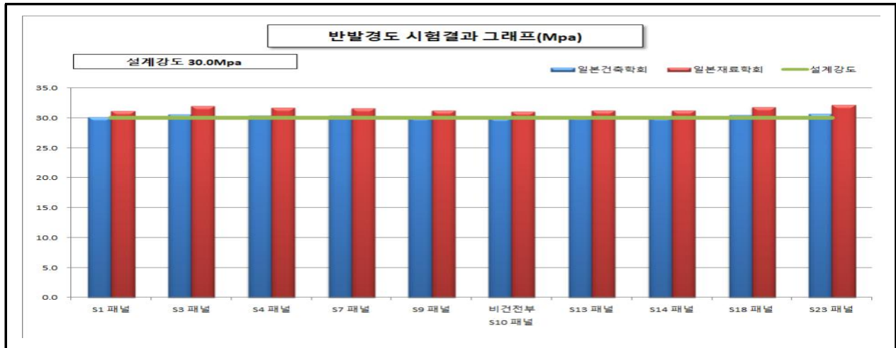
【그림 1.4.2】 반발경도시험 측정결과
